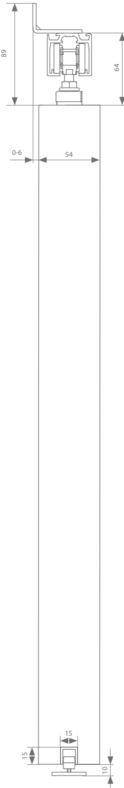
Muurbevestiging 54 mm
