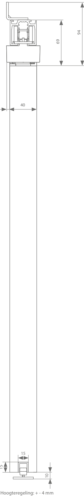
Muurbevestiging 40 mm
