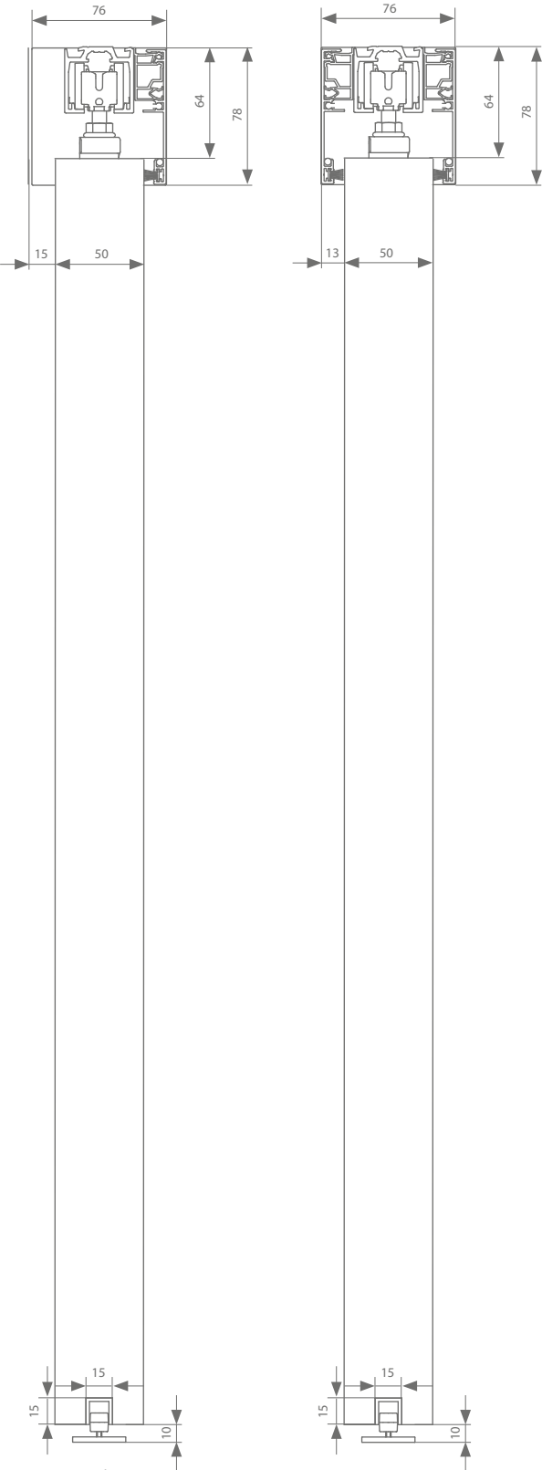
Plafondbevestiging 50 mm
