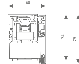
Muurbevestiging 44 mm
