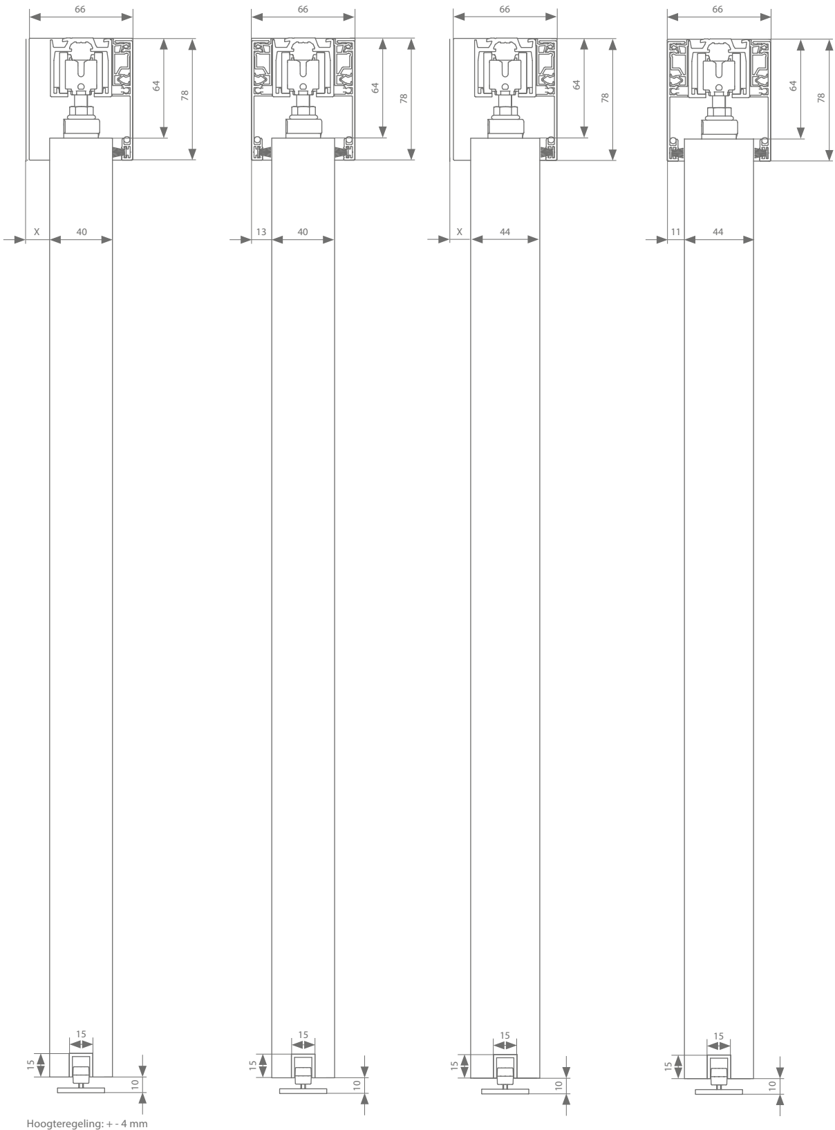
Plafondbevestiging 40 mm
