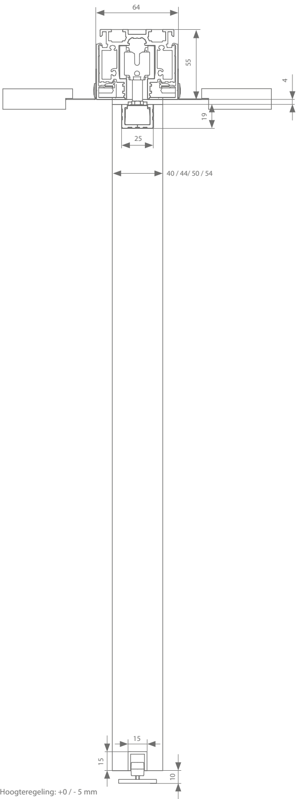
Voor systeemplafond (1+2)
