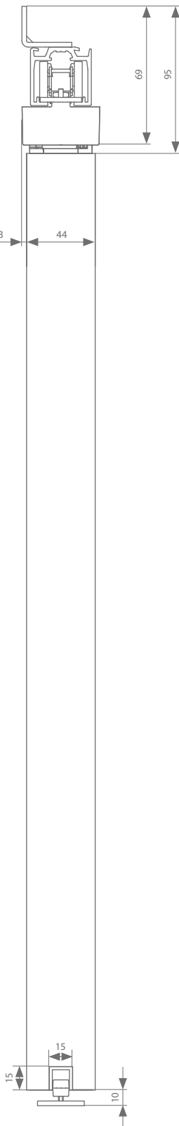
Muurbevestiging 44 mm
