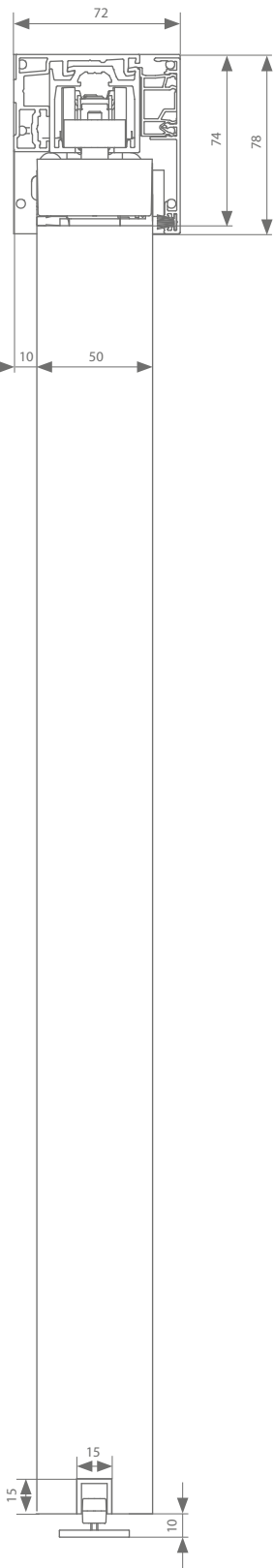
Muurbevestiging 50 mm
