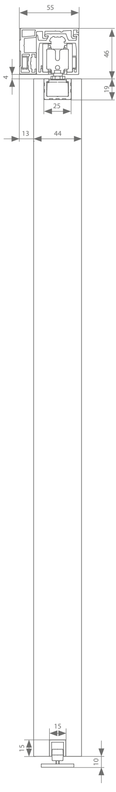
Muurbevestiging 44 mm
