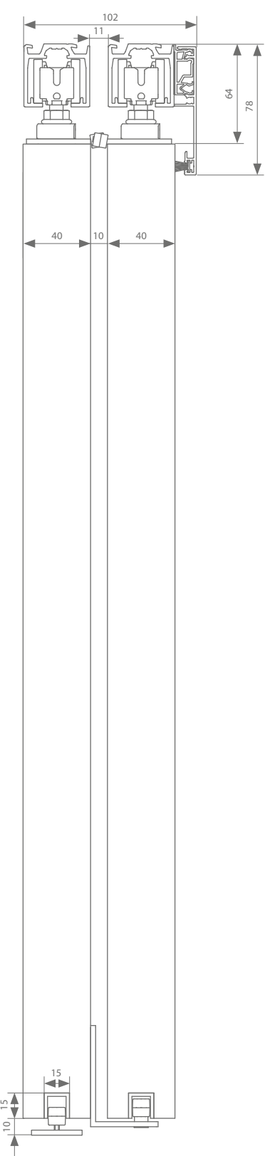
Parallelle plafondbevestiging 1
